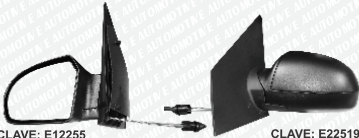
CLAVE: E12255 1FD225LL01 ESPEJO LATERAL CON CONTROL MANUAL NEGRO FORD FIESTA FIRST 03-10 NUM. ORIGINAL 1568916 DEPO 018-1217-15 IZQUIERDO L 22521 1VW225LL01
