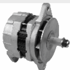
CLAVE: A03108 NO. PARTE: 19020310 ALTERNADOR DELCO REMY 22SI 12V 150A 3L
