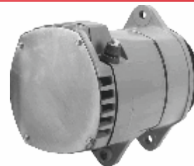
CLAVE: A48956 NO. PARTE: 48954 ALTERNADOR RCP DELCO 25SI 24V. 75A CANADA
